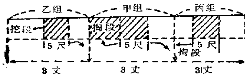
图 3 挖掘地道分段图棚顶式
