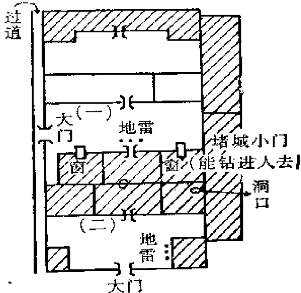
图 3 - 3 3 战斗院落
