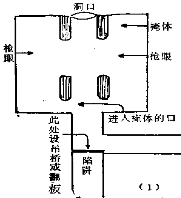
图18 脱险洞的构造
