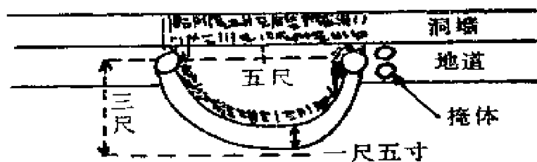
图16 卡口平面图
